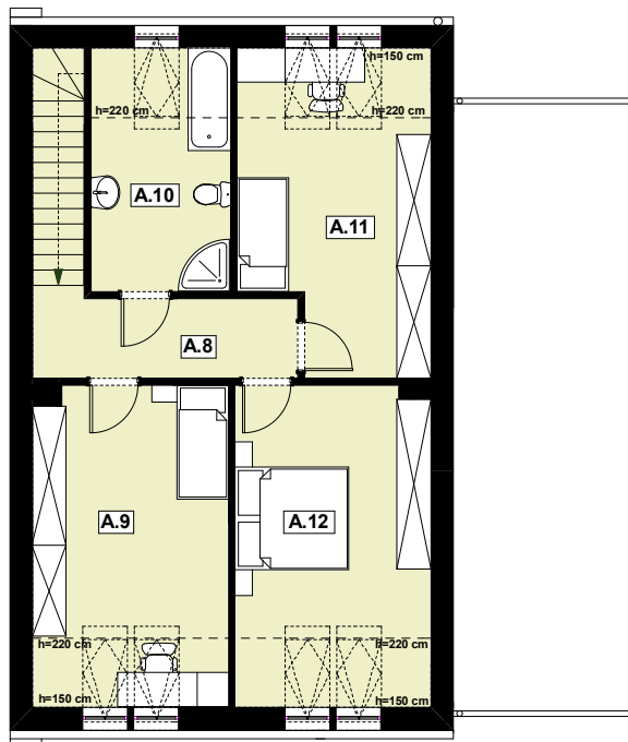
RZUT PODDASZA
