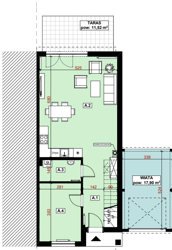
RZUT PARTERU
