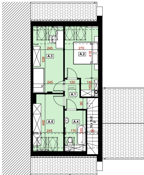
RZUT PODDASZA
