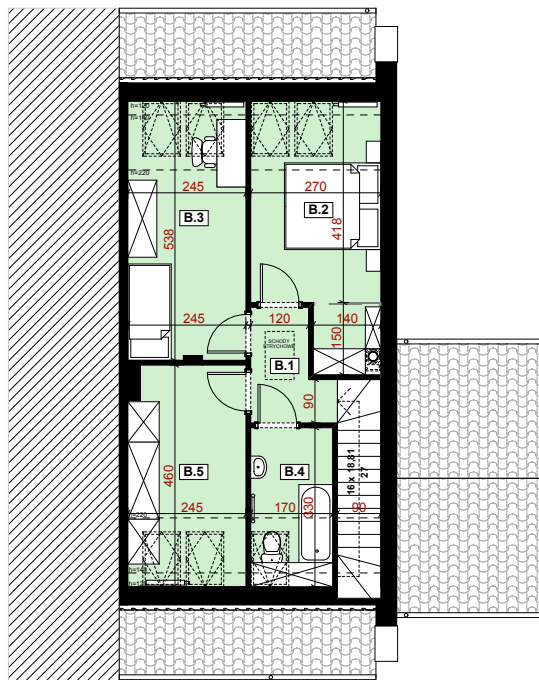
RZUT PODDASZA
