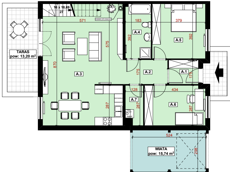
RZUT PARTERU
