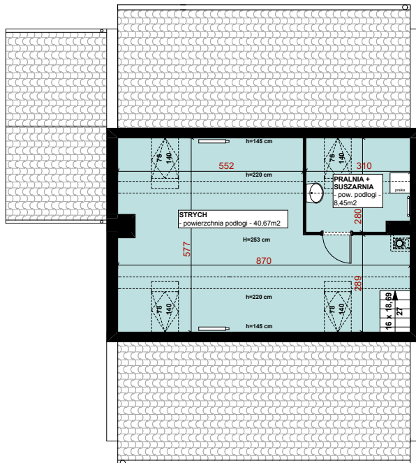
RZUT PODDASZA
